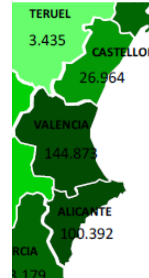
Parque BEV 2030
