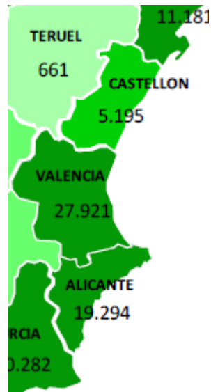
Parque BEV 2025
